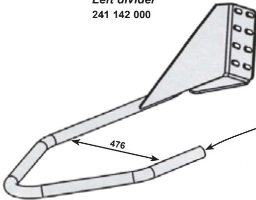
Diviseur gauche large Large left divider
