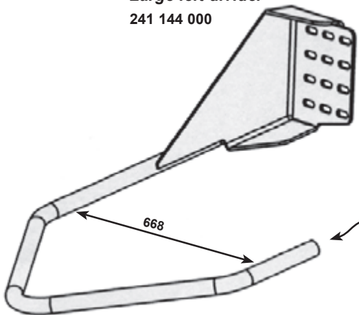
Diviseur gauche large Large left divider
